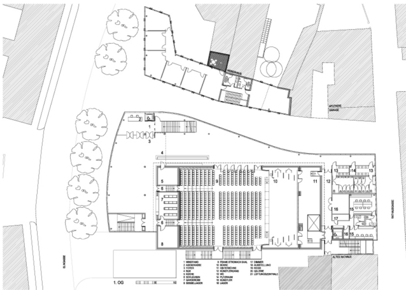
Grundriss OG1
