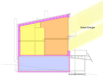
Raumzonen passiv solar
