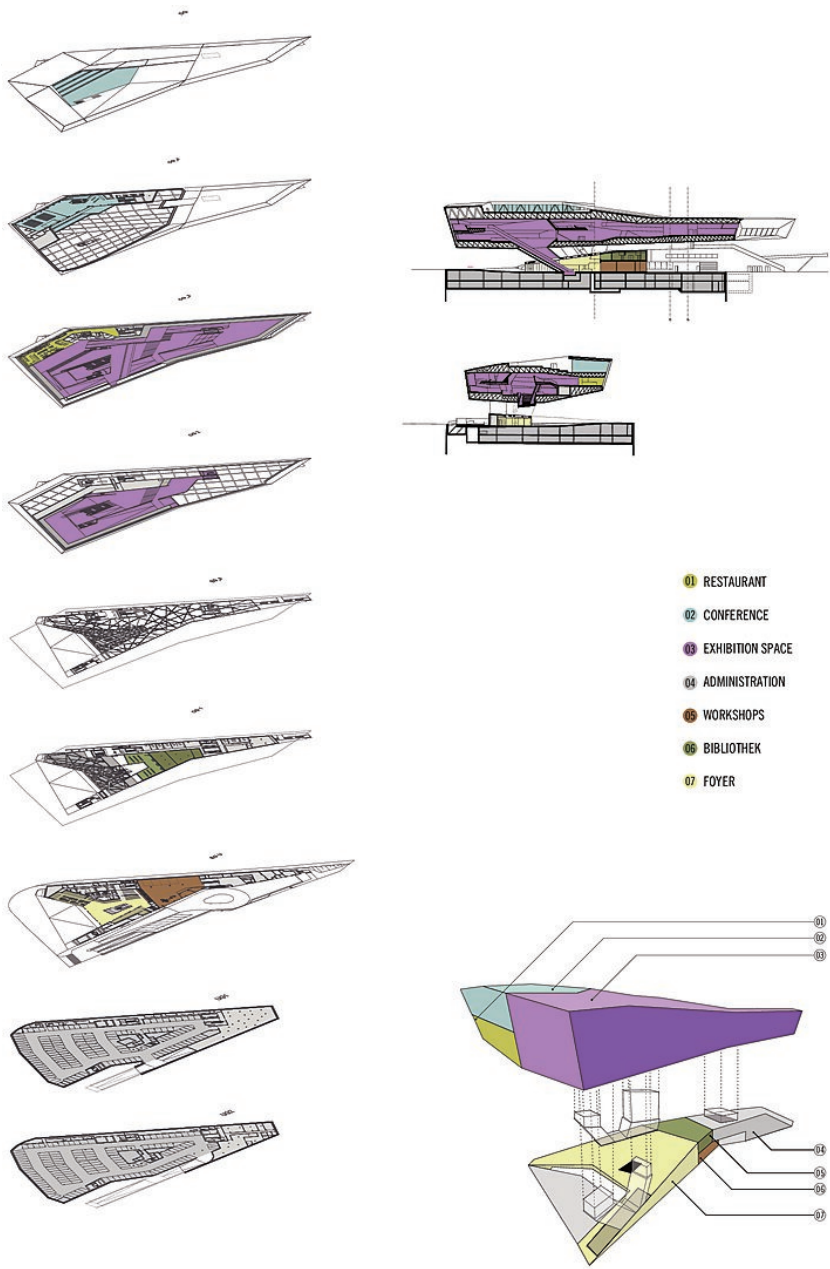
Raumprogramm Schnitt
