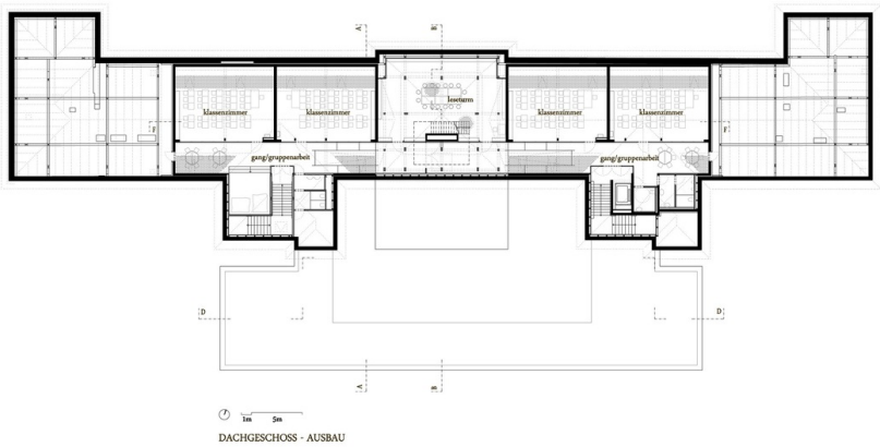
Grundriss DG
