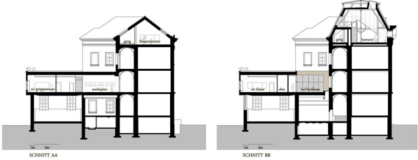
Querschnitte
