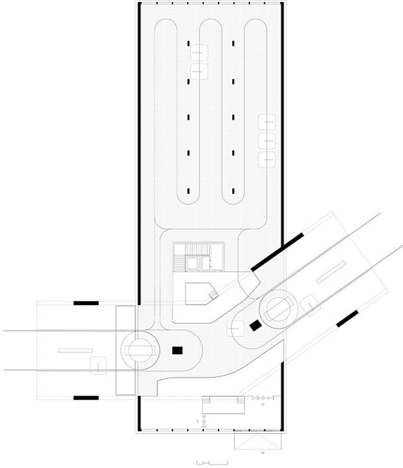
grundriss mittelstation 1:250
