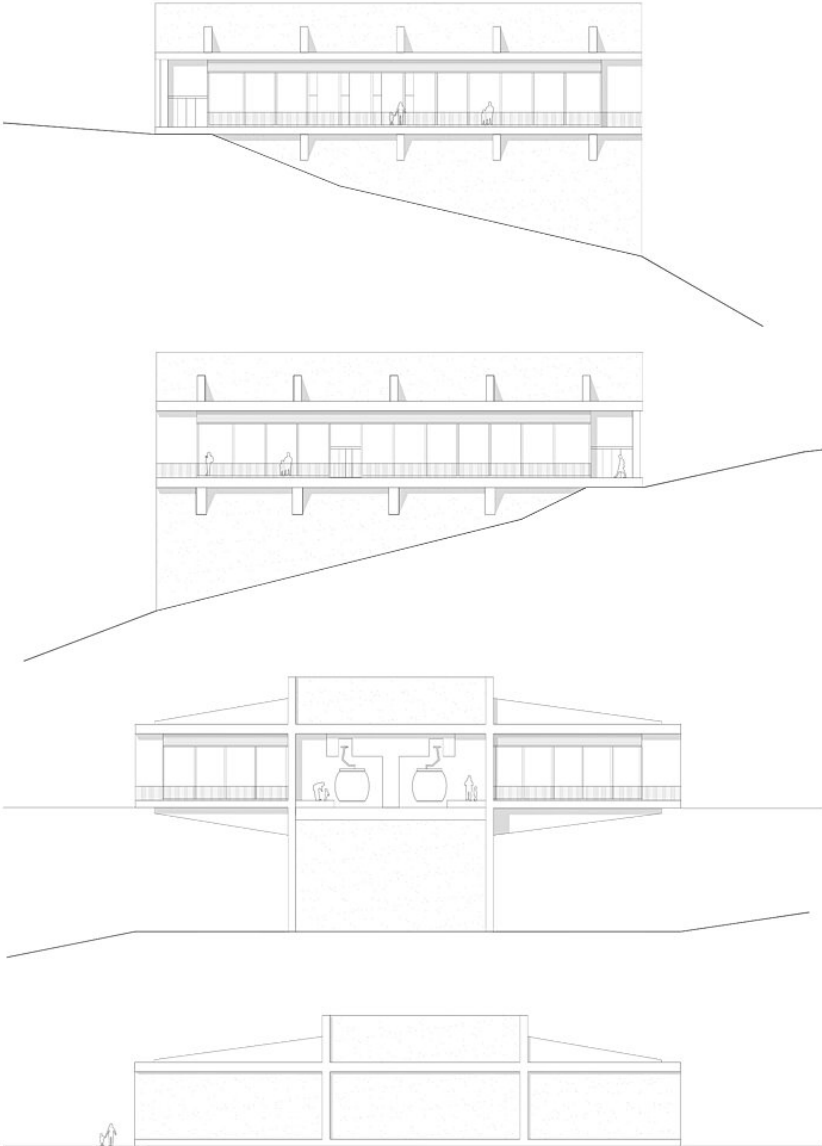
ansichten bergstation 1:250
