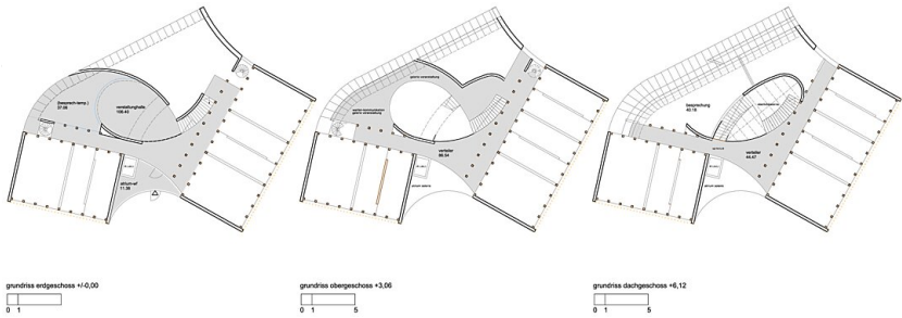
Grundrisse
