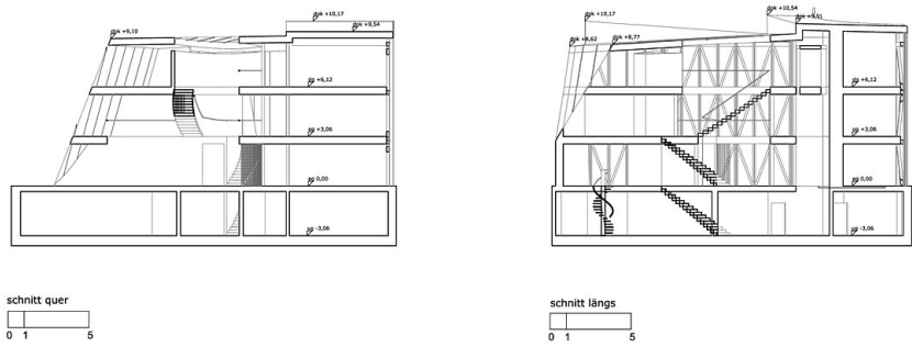
Schnitte
