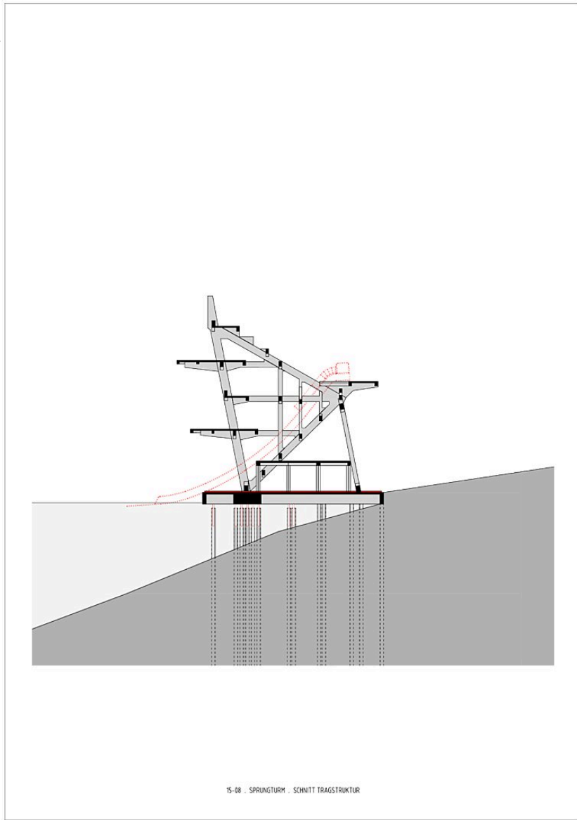
Schnitt Tragstruktur
