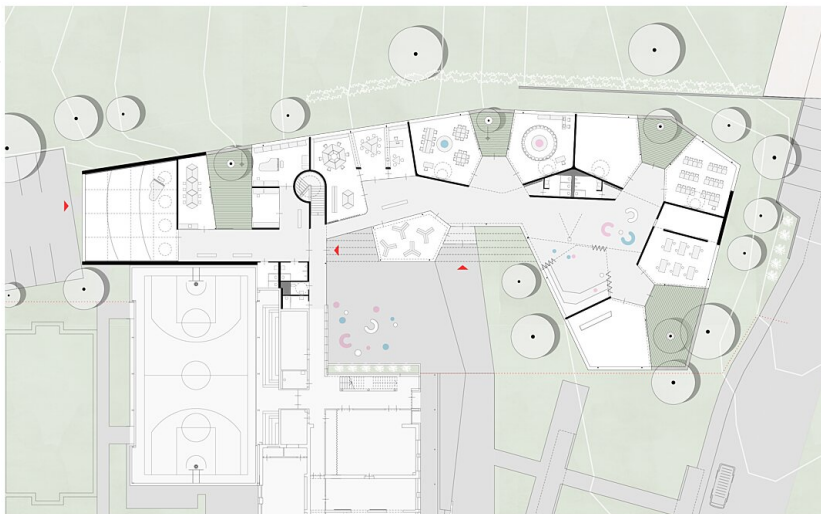
Grundriss EG
