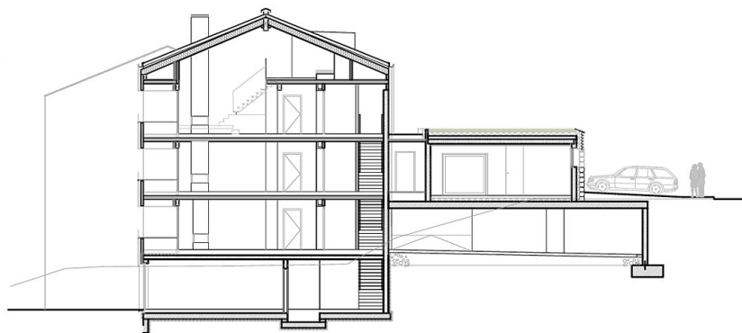
Querschnitt 2
