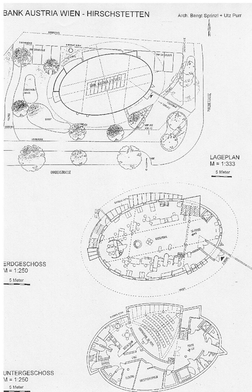
Lageplan/Grundrisse
