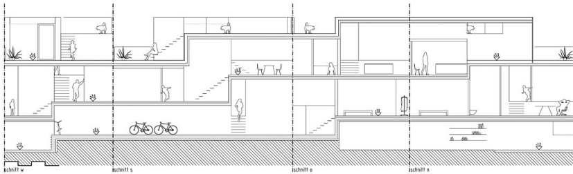
Schnitte
