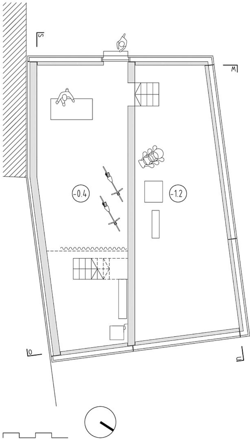
Grundriss UG
