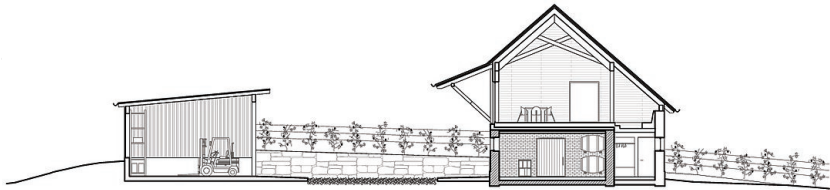
LÄNGSSCHNITT M 1:200
