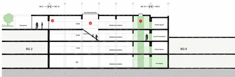
Schnitt M 1:200
