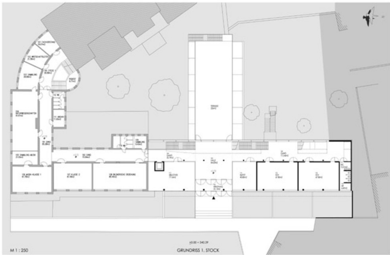
M 1 : 250 GRUNDRISS I. STOCK HLW / FW STADT HAAG • ERWEITERUNG UND SANIERUNG SOWIE ERRICHTUNG EINES TURNHALES • ARCHITEKTURBÜRO SCHWALM-THIESS & GRESSENBAUER • 30. NOVEMBER 2000 • ENTWURF
