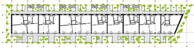
Grundriss OG
