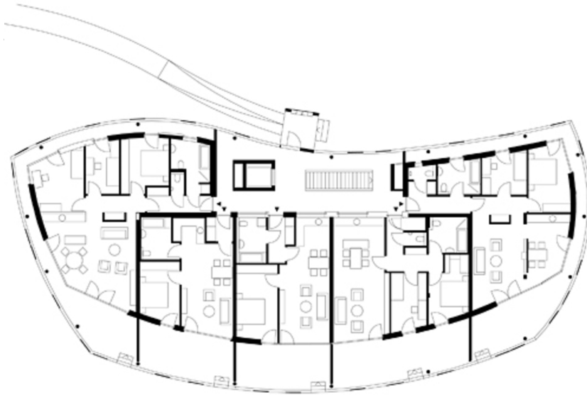
6 Erdgeschoss Haus C
