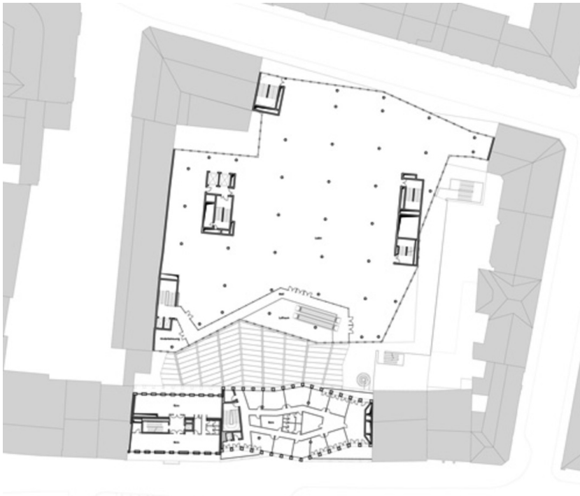
Grundriss OG4
