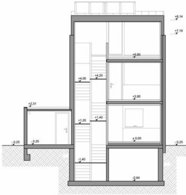
schnitt b-b
