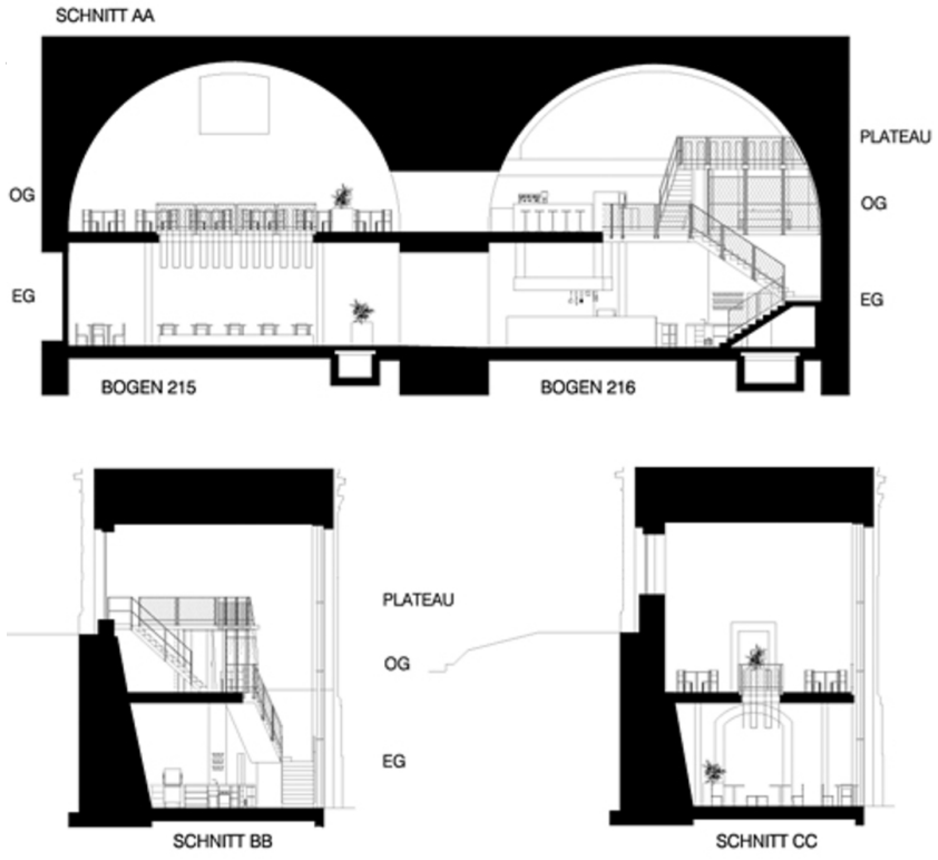
Schnitte
