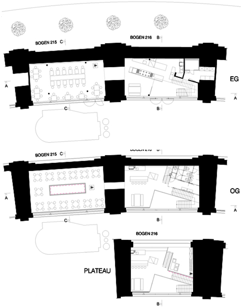
Grundriss
