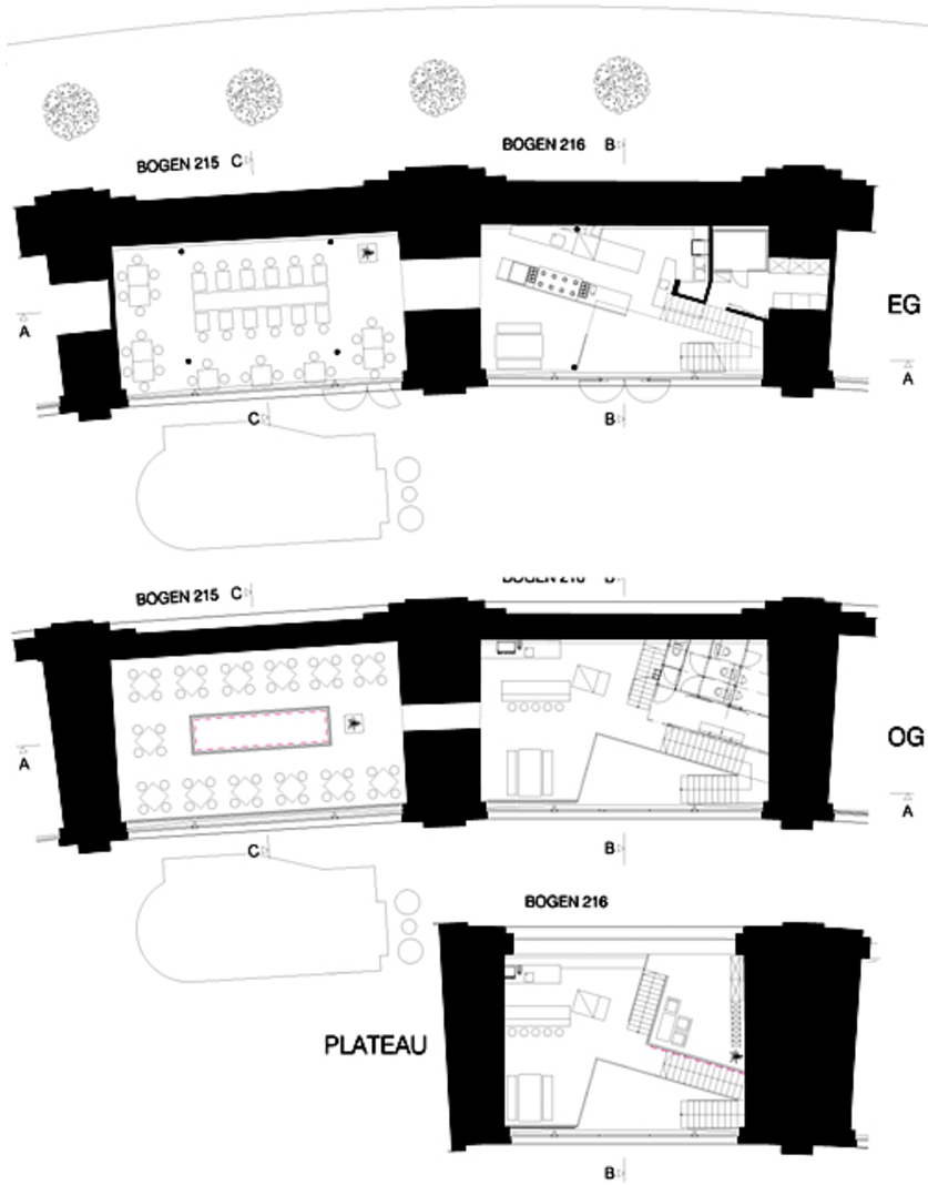
Grundriss
