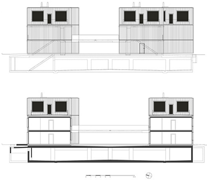
Schnitt
