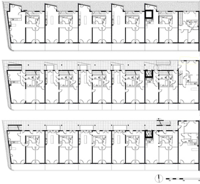
Grundriss OG
