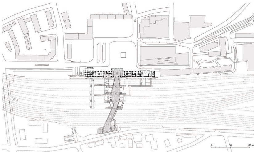
Grundriss Passagenebene
