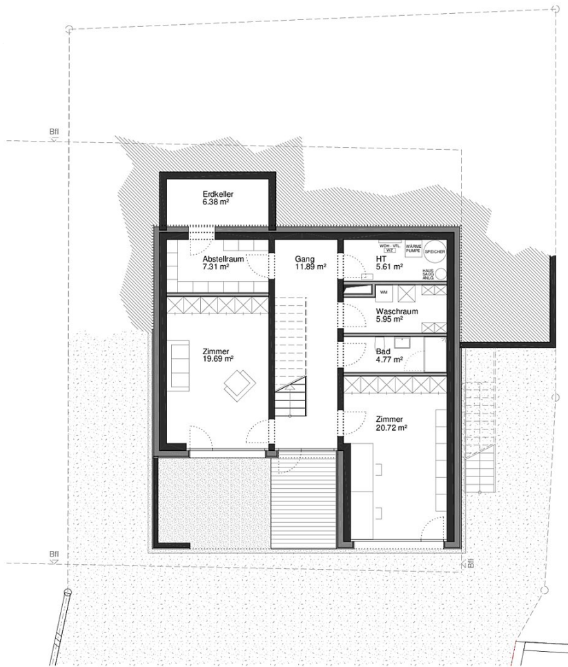
Grundriss UG
