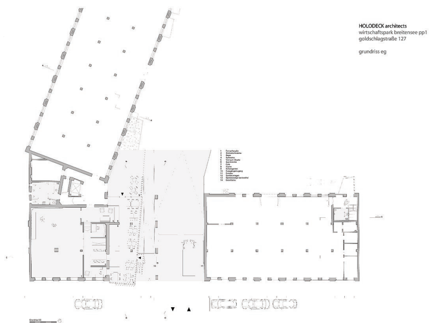
Grundriss EG
