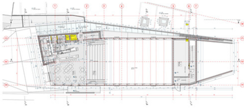
Grundriss EG
