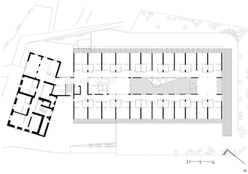
Grundriss OG
