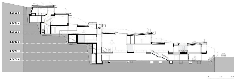
Schnitt B
