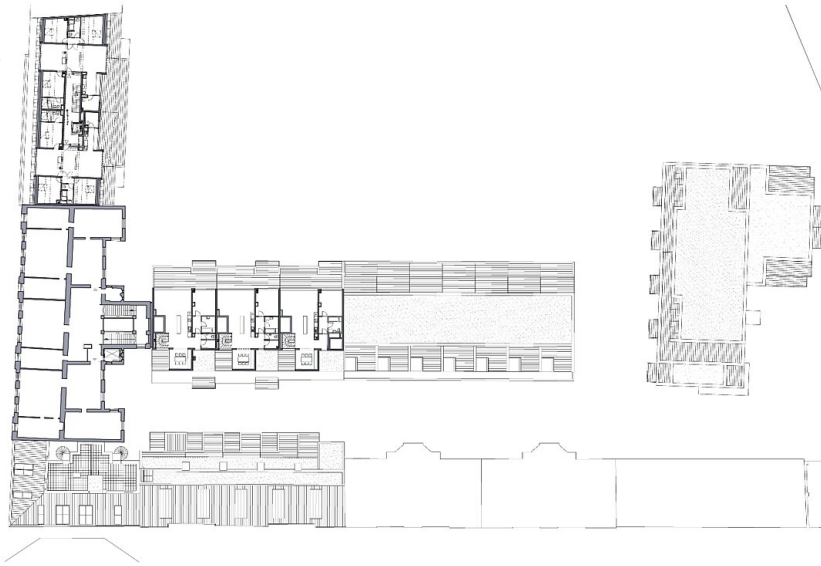
Grundriss 2. DG
