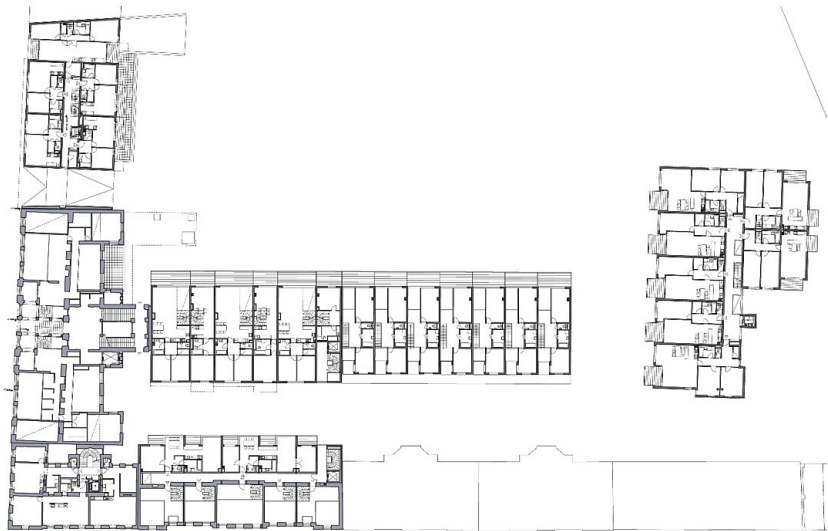
Grundriss 1. OG
