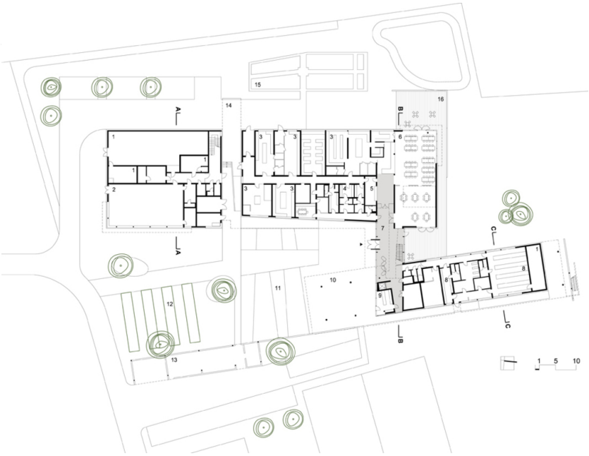
Grundriss EG
