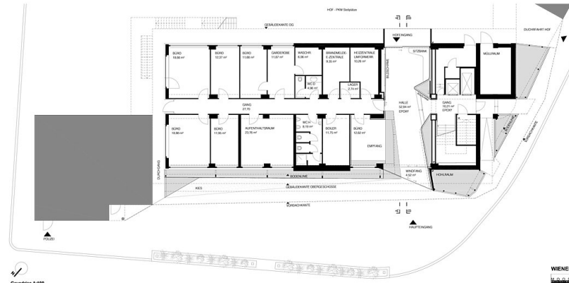
Grundriss 1:100
