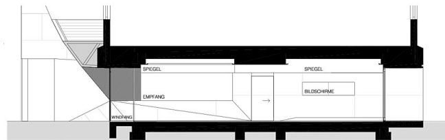
Schnitt A-A 1:100
