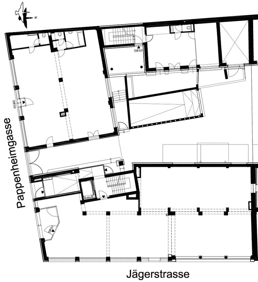
Erdgeschoss
