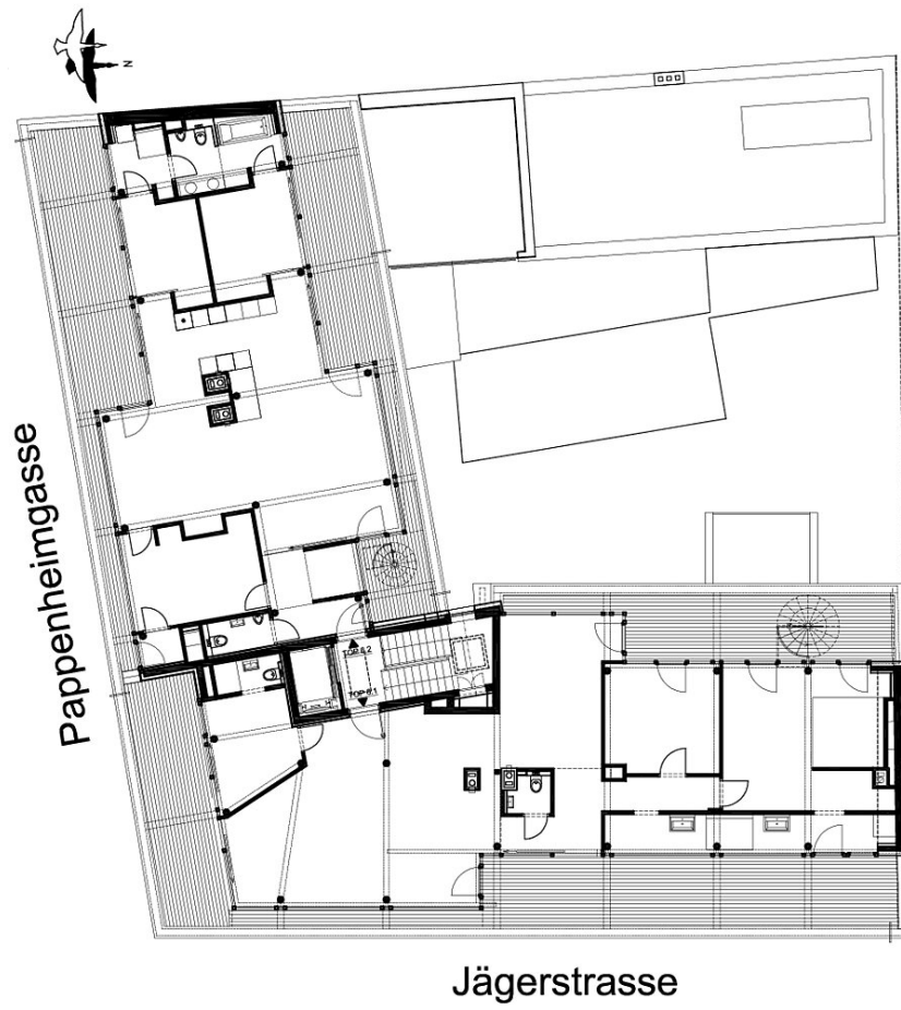
Dachgeschoss
