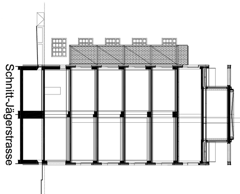
Dachgeschoss
