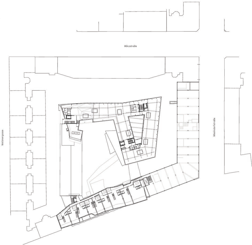
grundriss e2
