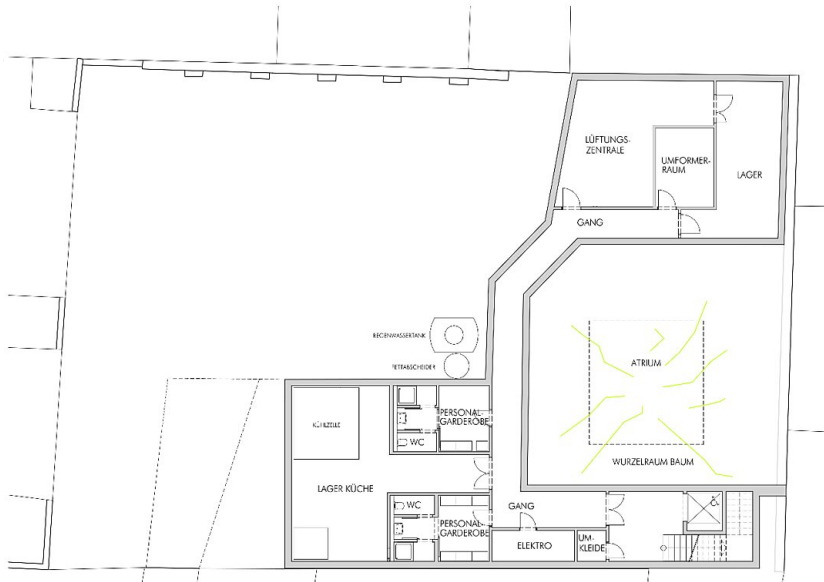
Grundriss Kellergeschoss
