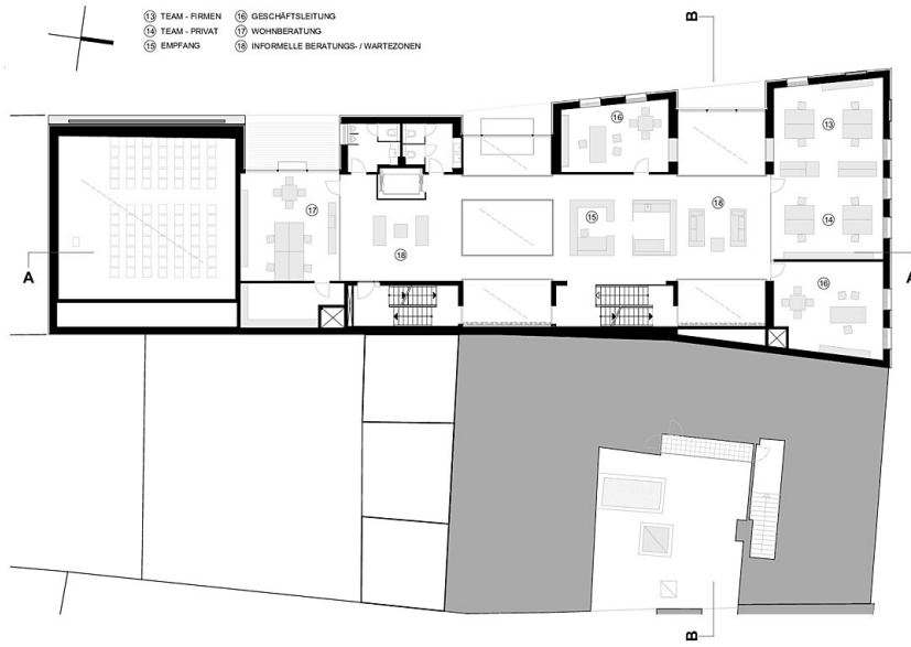
Grundriss Obergeschoss
