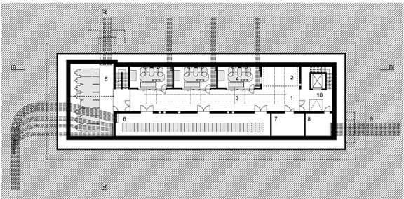
Grundriss 2. Untergeschoss (G02)
