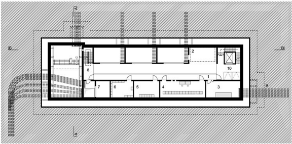
Grundriss 1. Untergeschoss (G01)
