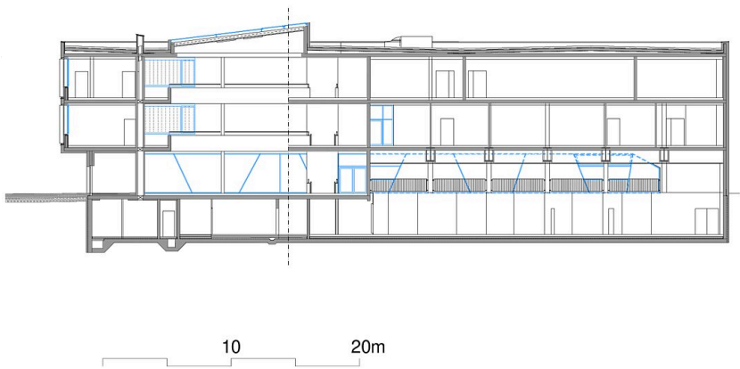
Schnitt Kopfbau
