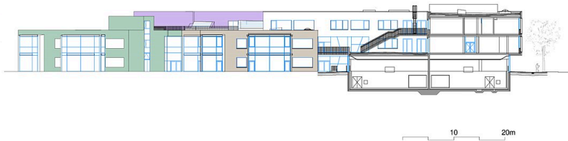
Ansicht SW und Querschnitt Kopfbau
