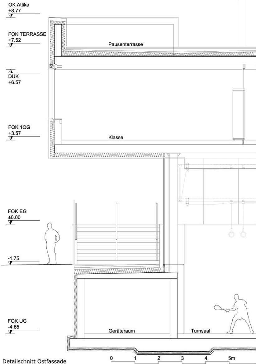
Detailschnitt Ostfassade
