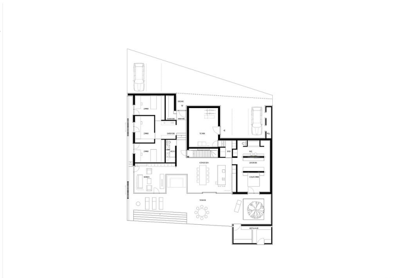
M 1:200 ERDGESCHOSS
