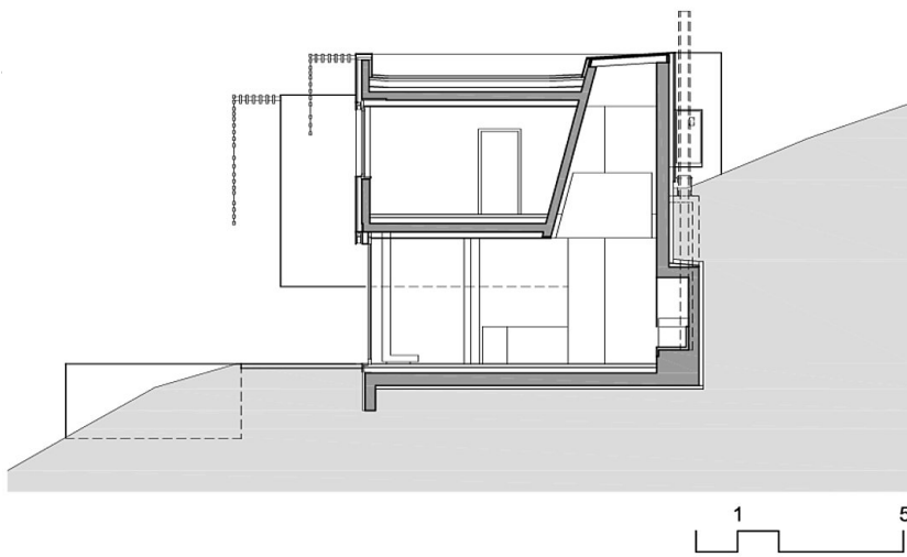
Querschnitt 2
