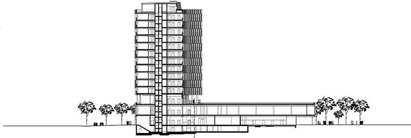
Schnitt N-S
