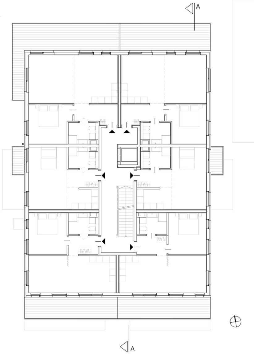
Grundriss OG1
