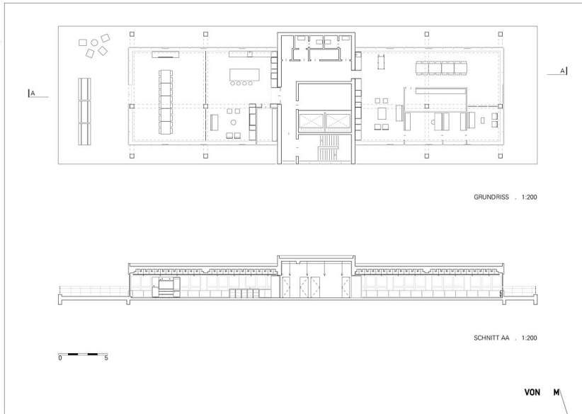
Grundriss & Schnitt
