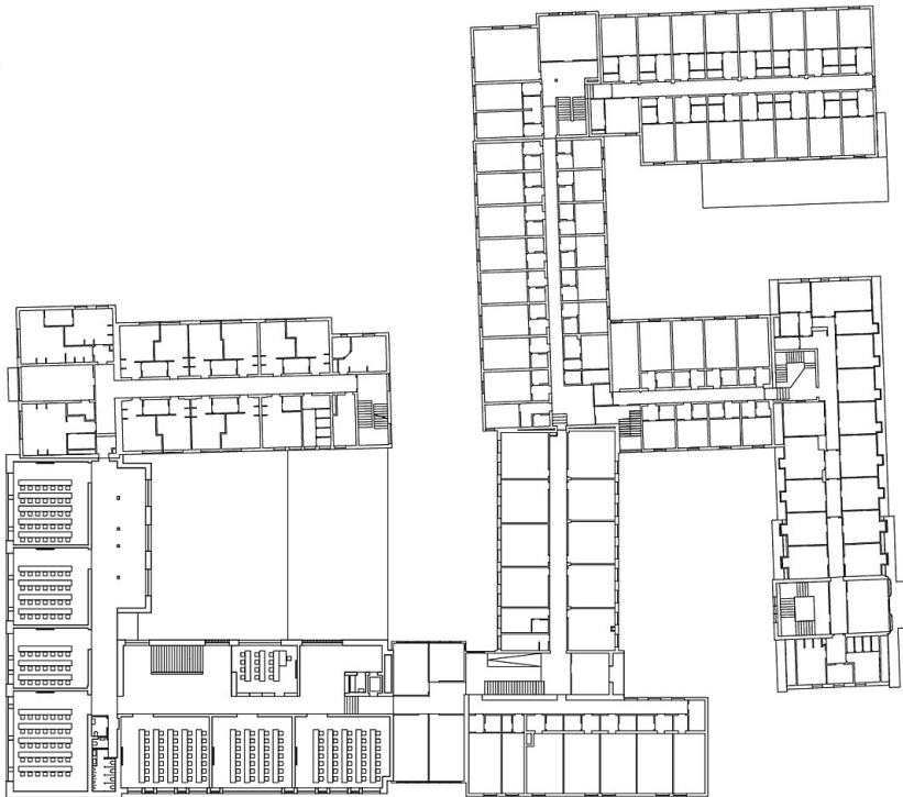
Grundriss OG2
