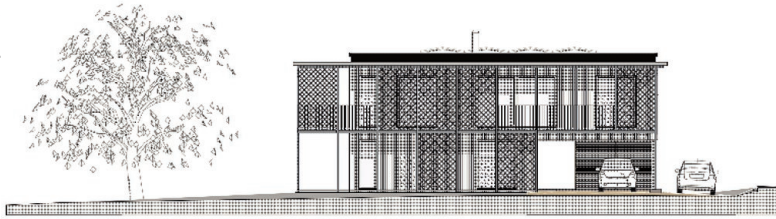
ANSICHT SÜD - WEST
