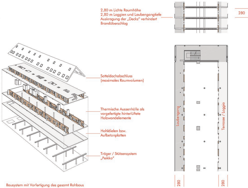
Bausystem mit Vorfertigung des gesamt Rohbaus
