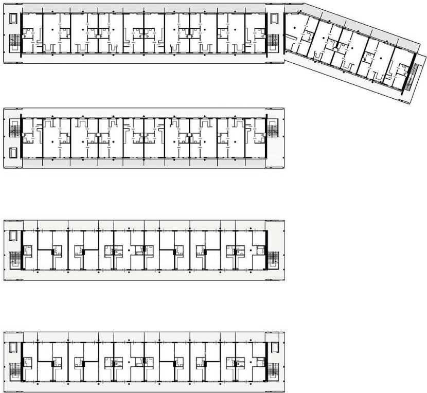
OG1 Grundriss OG1
