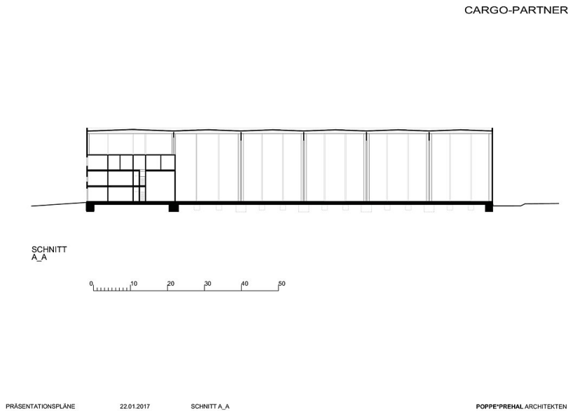
Schnitt AA
