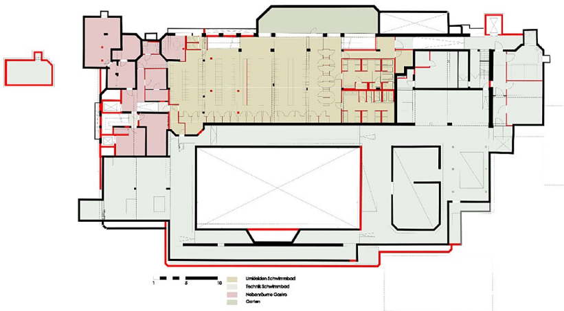
Grundriss UG
