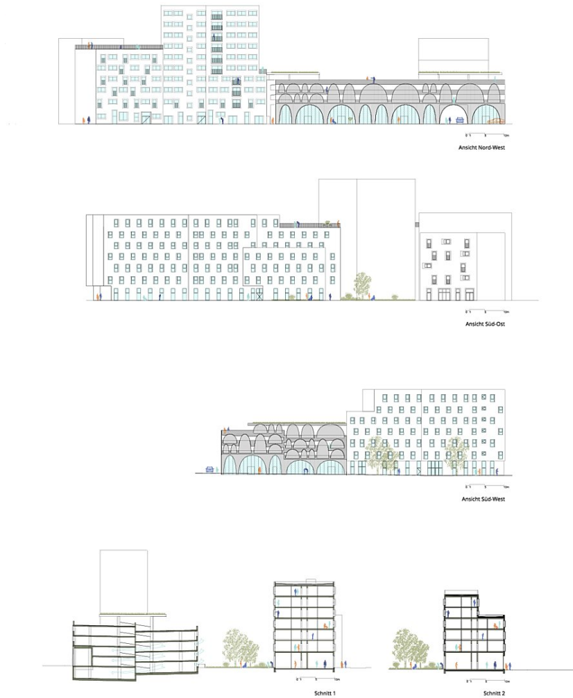
Ansichten, Schnitte
