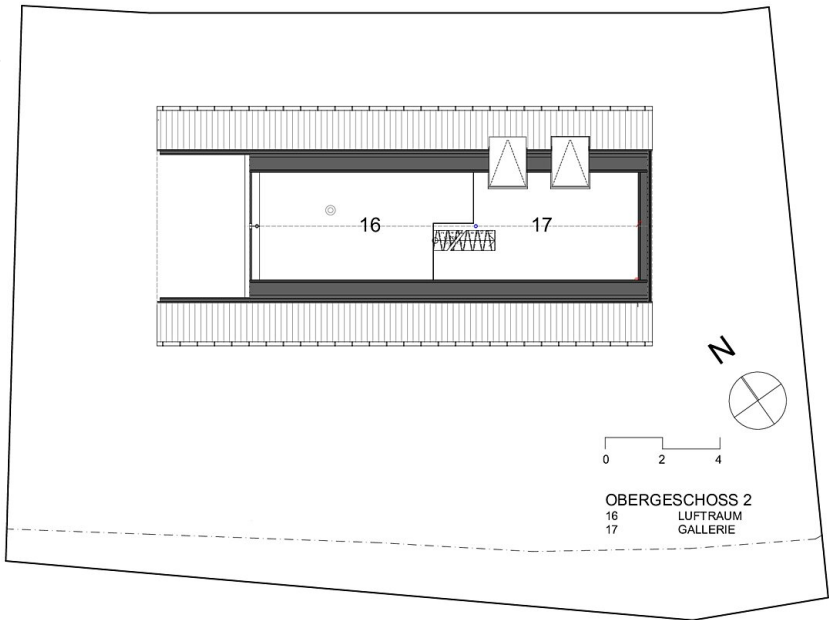
Grundriss OG 2
